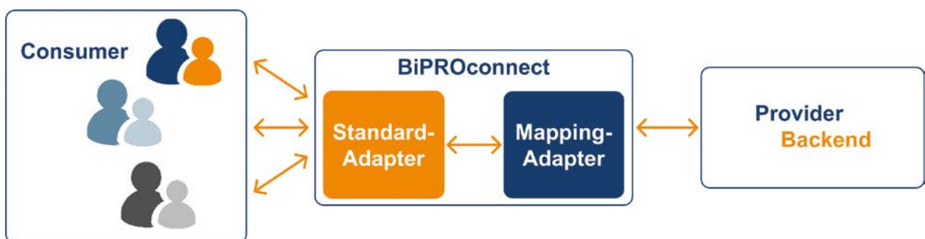
BiPROconnect: Nutzung auf Providerseite
